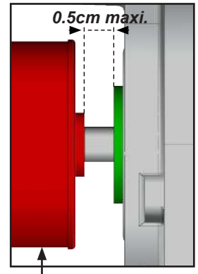
TOURILLON
